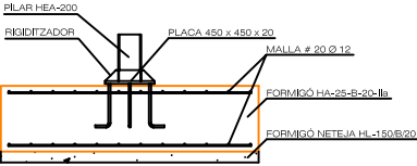
DETALL SABATA TIPUS 1 (S1-S7 / S24-S30)
