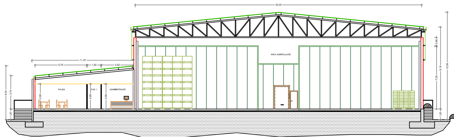
SECCIÓ A-A'
