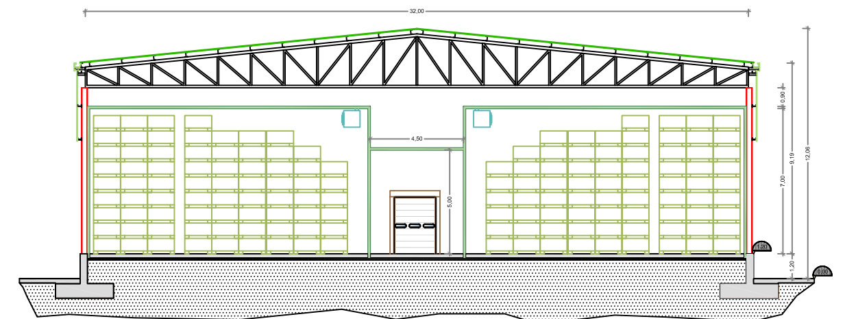
SECCIÓ A-A'
