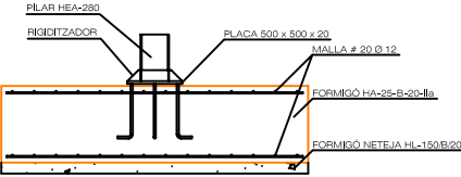
DETALL SABATA TIPUS 2 (S8-S23 / S31-S46)
