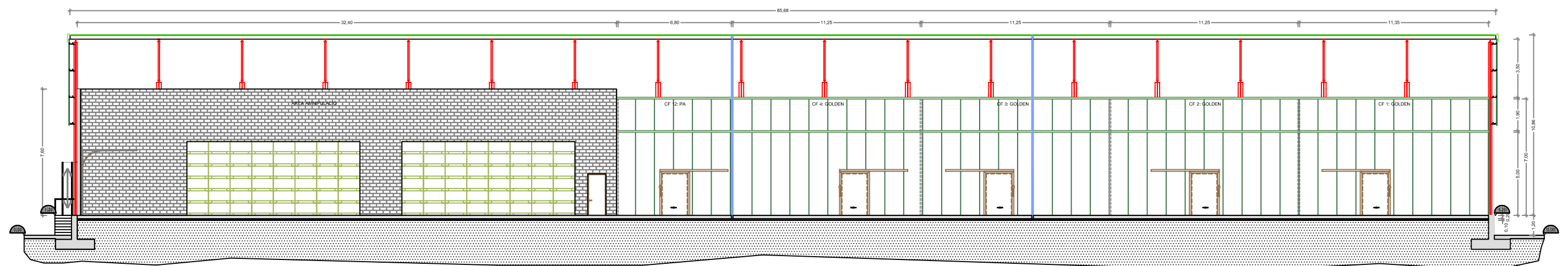
SECCIÓ C-C'
