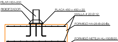
DETALL SABATA TIPUS 3 (47-52)
