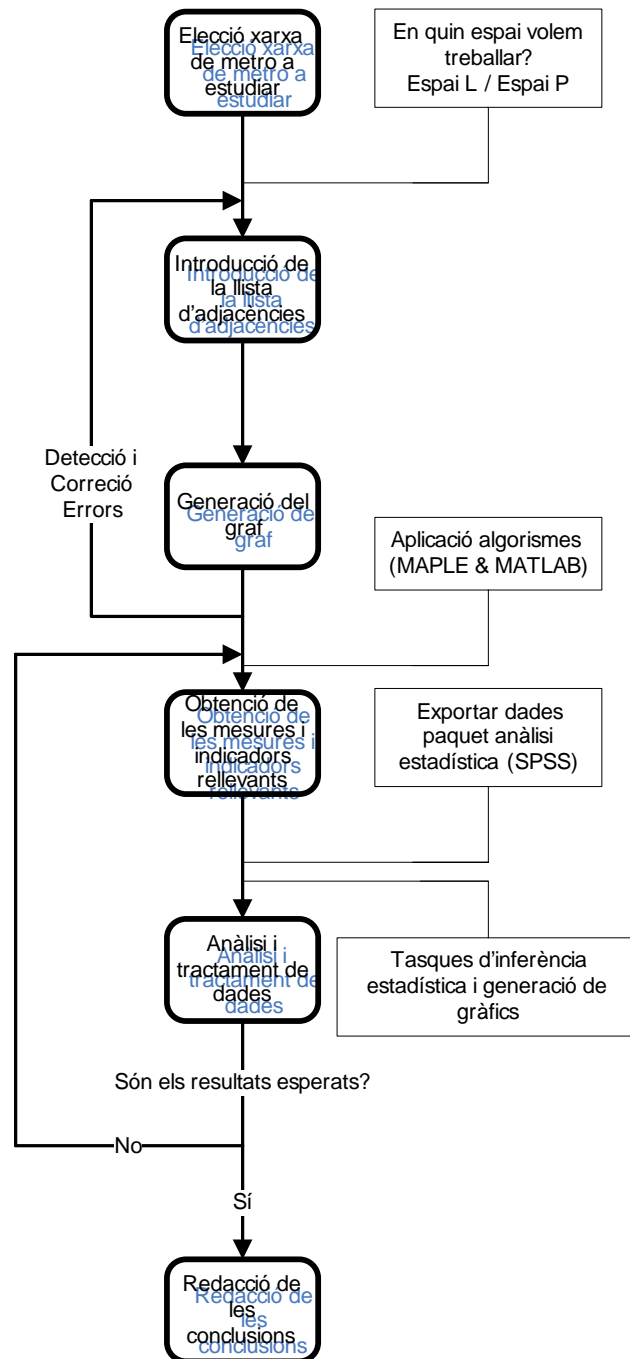
Figura 3. Diagrama de flux detallat del procés seguit des de la inicial introducció de dades d'una determinada xarxa fins a la corresponent anàlisi i tractament de mesures i indicadors obtinguts.
