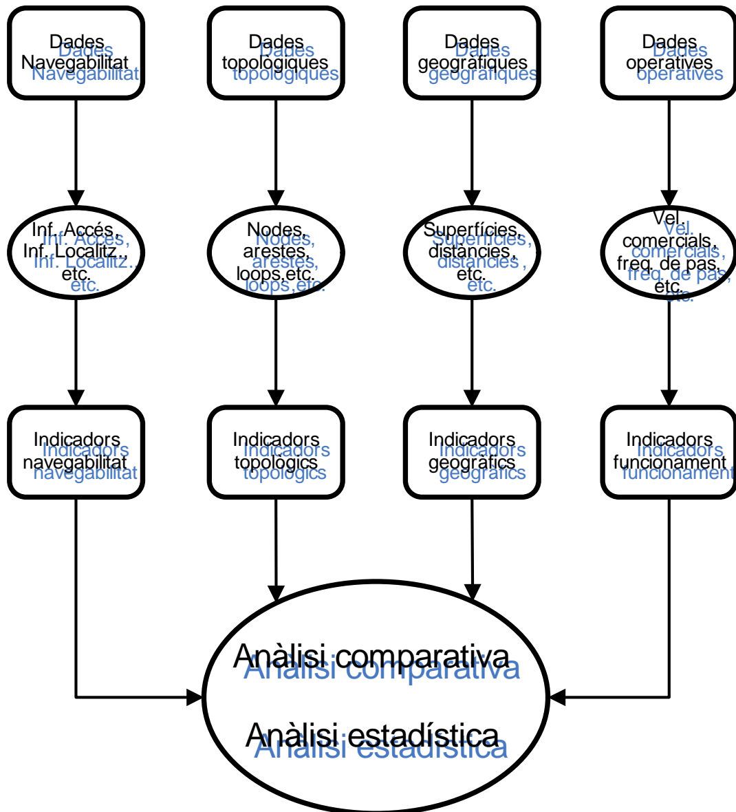
Figura 1. Segons la tipologia de les dades de que es disposi es pot enfocar l'anàlisi de les xarxes des d'una perspectiva o una altra. El nostre estudi se centra en l'anàlisi d'indicadors topològics i de navegabilitat de les diferents xarxes analitzades.
