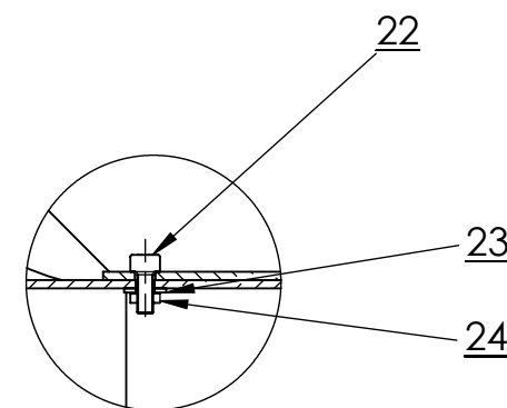
C (1 : 2)
