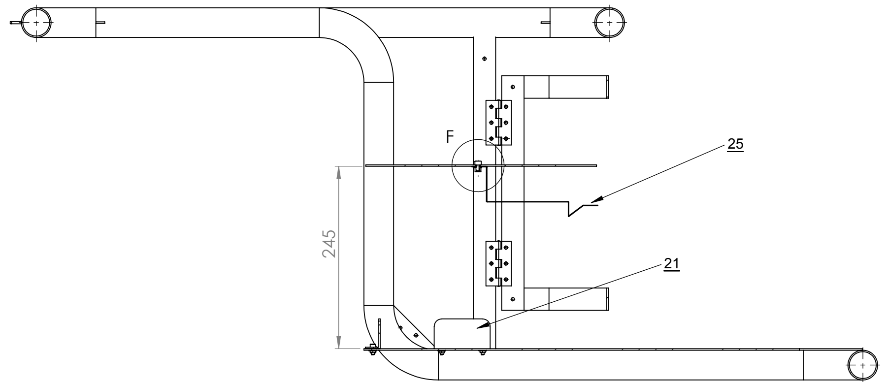
E-E (1 : 5)
