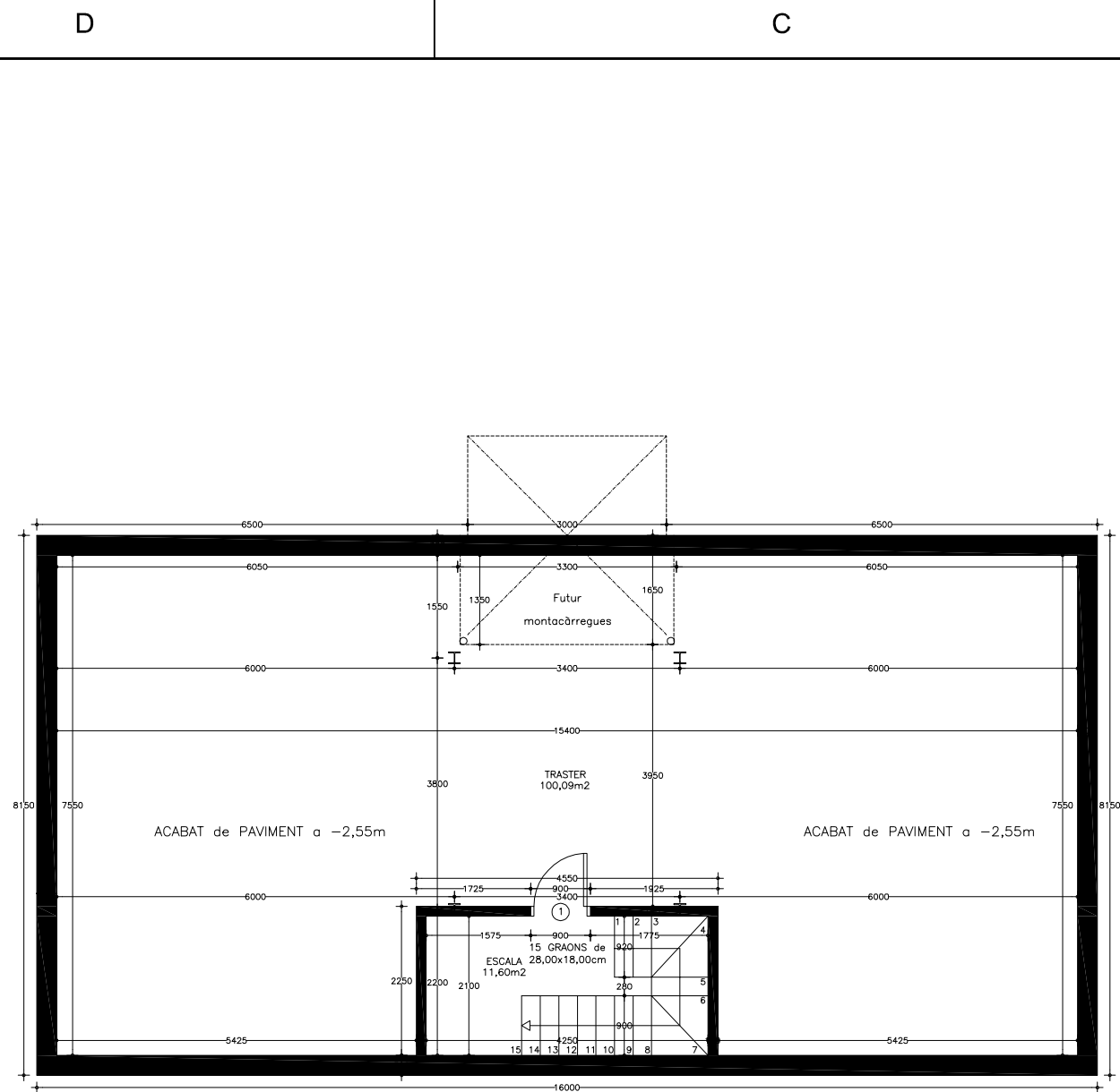
PLANTA SOTERRANI
