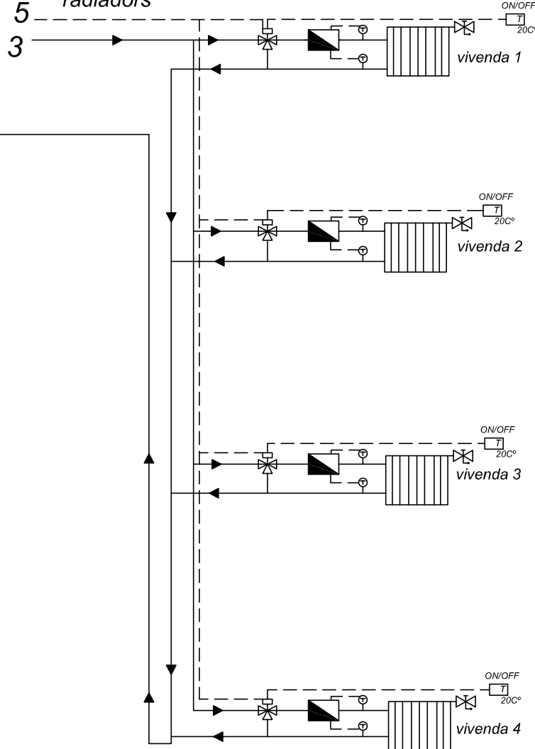
Distribució radiadors
