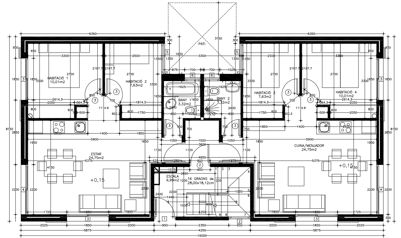
PLANTA BAIXA
