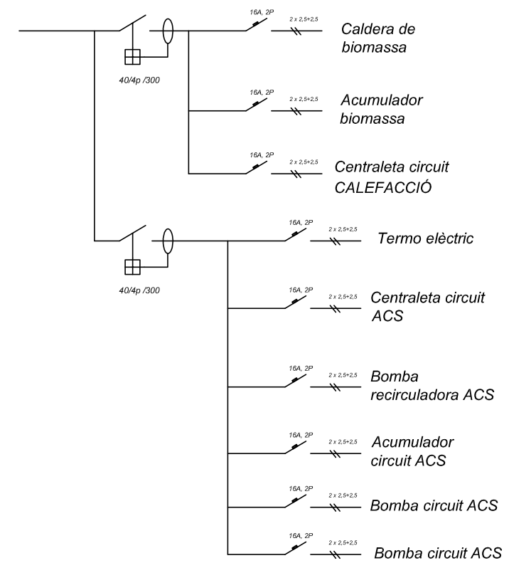
Esquema elèctric
