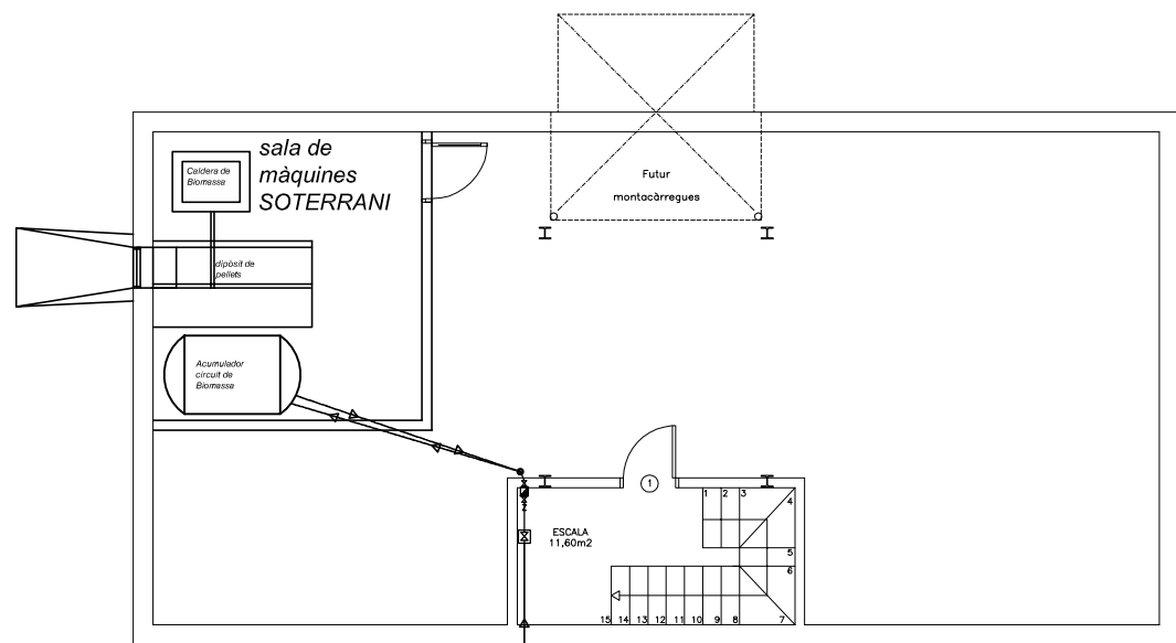
PLANTA SOTERRANI
