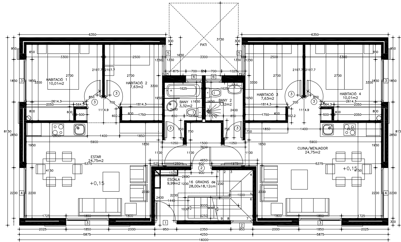
PRIMERA PLANTA
