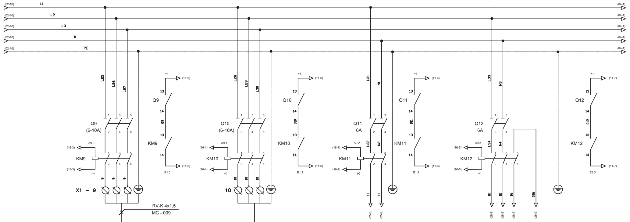
VEURE A PAG. 25 DW-PM-03 DOSIFICADORA HIPOCLORIT
