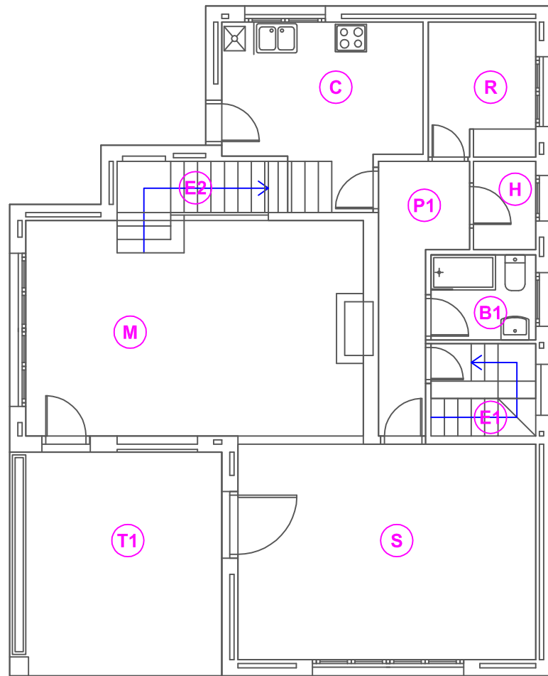
Planta Baixa H=2.80 m
