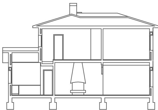
Secció D-D
