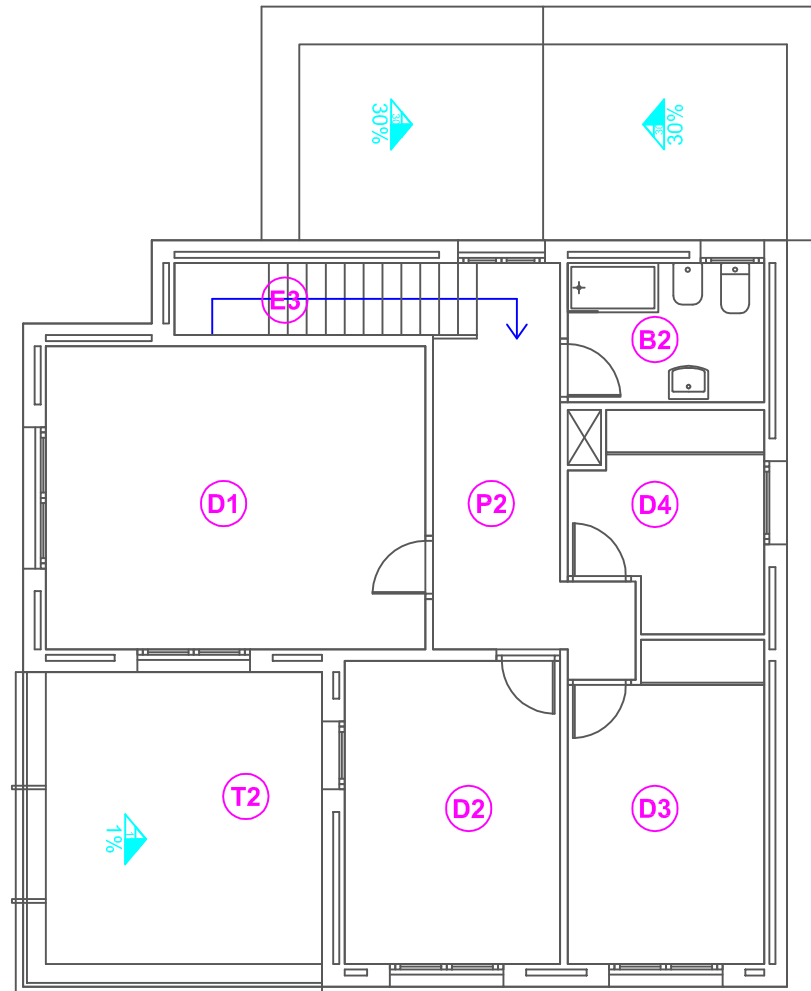
Planta Primera H=2.70 m
