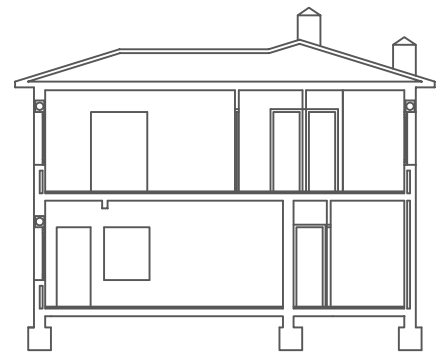
Secció C-C
