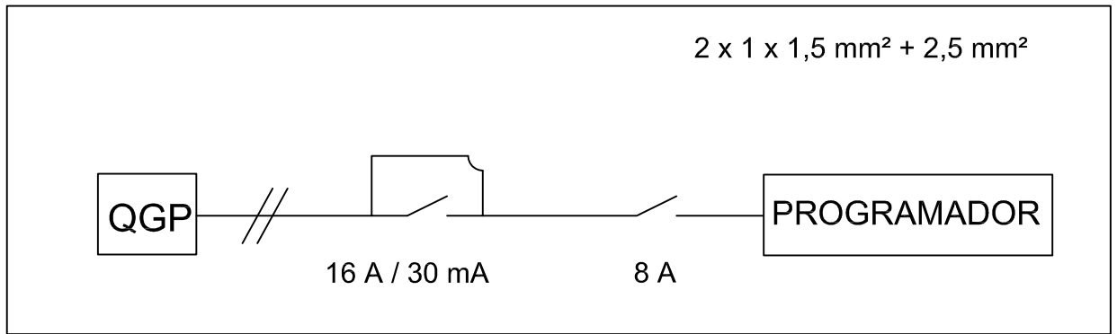
Esquema unifilar de la línia del programador
