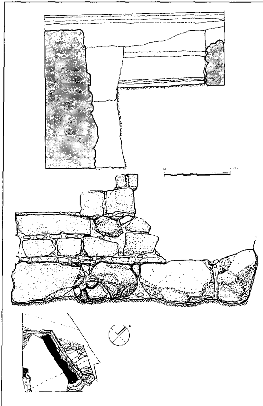
Làm. 3.- Alçat i secció del parament interior de la muralla augustina en l'angle nord.
