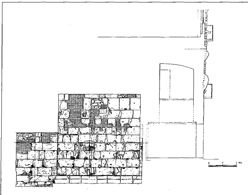
Làm. 10.- Alçat de la muralla del c/ 1 i Arc de Sant Ramon del Call,5
