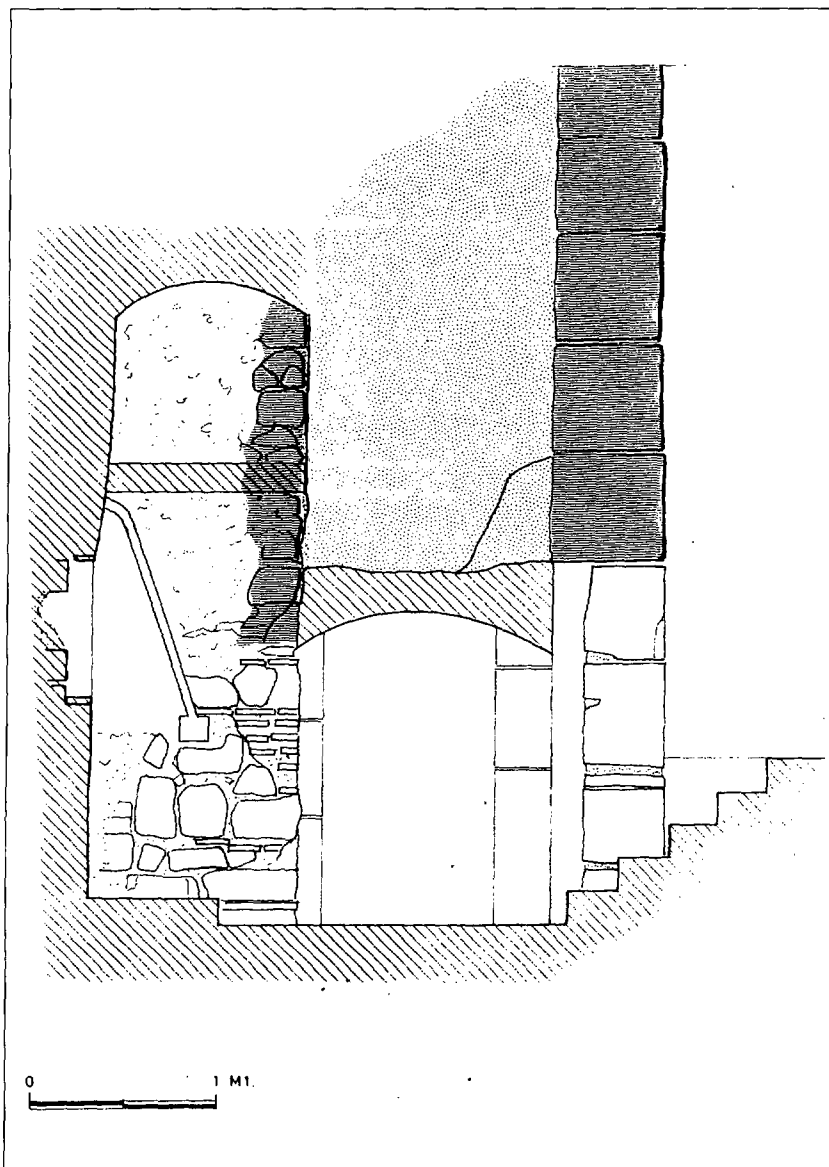
Làm. 7.- Secció de les dues muralles al c. Avinyó 19
