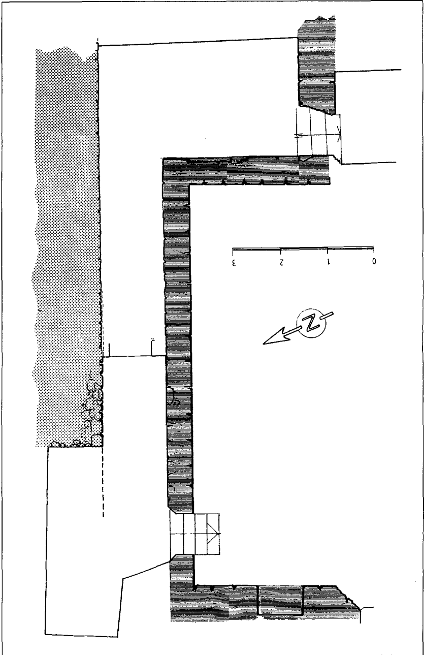
Làm. 6.- Planta del sector de muralla del c. Avinyó 19
