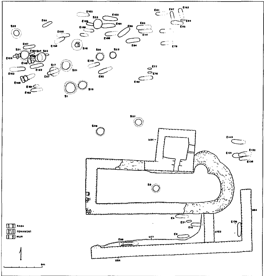
Figura 3.- Planta de la fase III: l'església romànica i la sagrera (dibuix, Jordi ROIG i BUXÓ, 1994).
