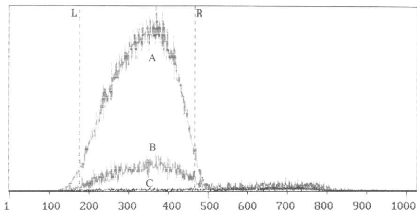
Fig. 2. Espectre d'emissió 6 obtingut de l'anàlisi de la mostra. L i R marquen els límits de la finestra de comptatge. A, B i C són, respectivament, l'espectre d'un àcid oxàlic actual, l'espectre de la mostra i l'espectre del fons del comptador.
