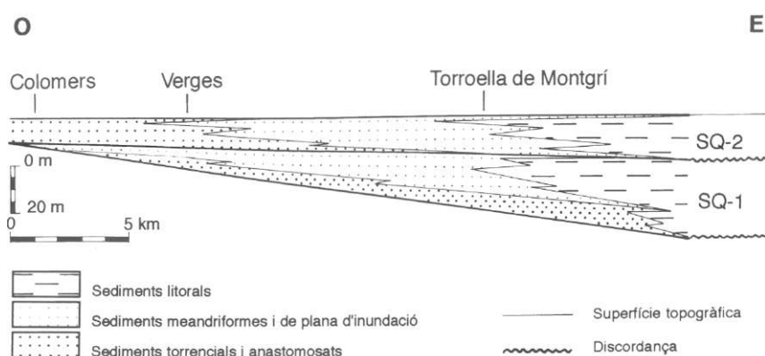
Figura 2. Esquema de les seqüències de rebliment de la Plana de Ter. (Modificat de Montaner et al. 1995).
