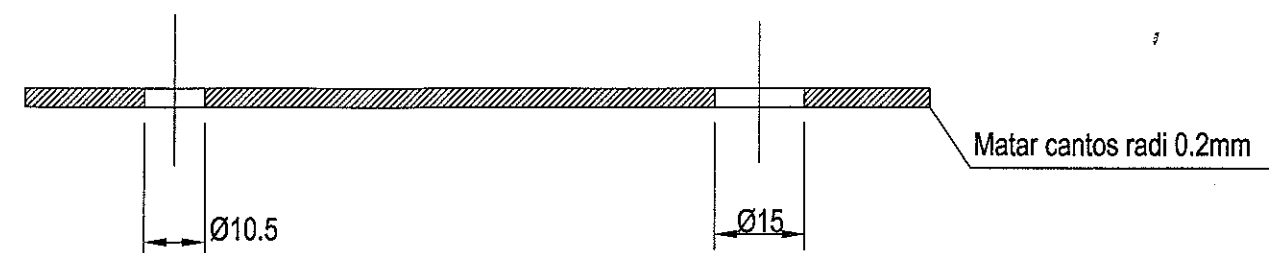
Tall A-A
