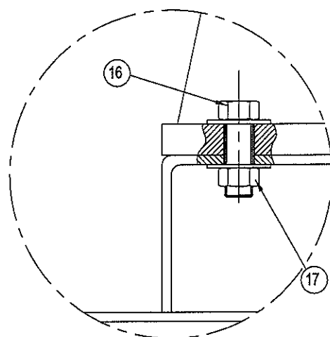
DETALL A
