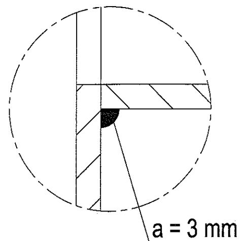
Detall A
