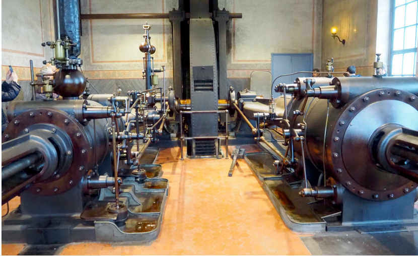
Fig. 8. Màquina de vapor de la fàbrica Burés d'Anglès.
