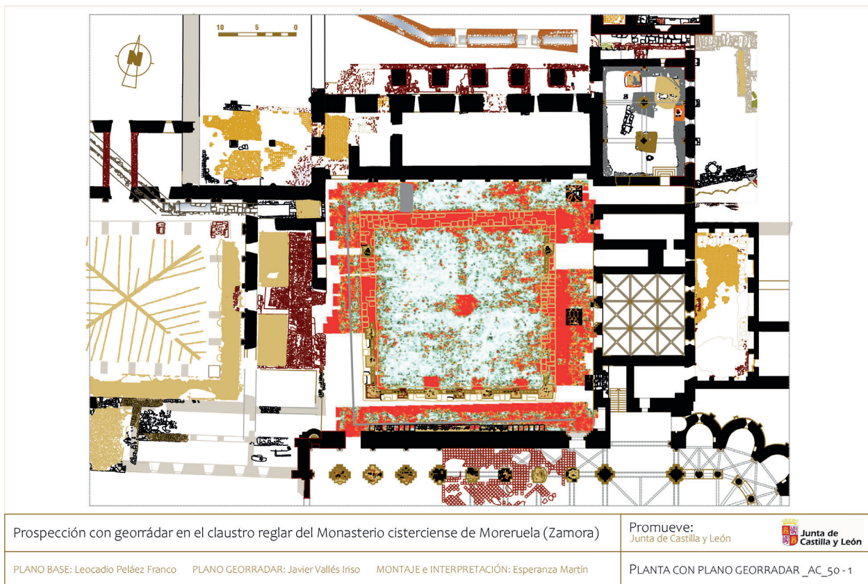
Figura 24. «Mapa» del georradar 3D en el claustro reglar del monasterio de Moreuella, de J. Vallés y E. Martín (CAI de ciencias de la Tierra y Arqueometría UCM), en noviembre de 2020, sobre plano de Leocadio Peláez. En rojo grueso, cimentaciones del claustro medieval y moderno; círculo central de la posible fuente y otras «perturbaciones».
