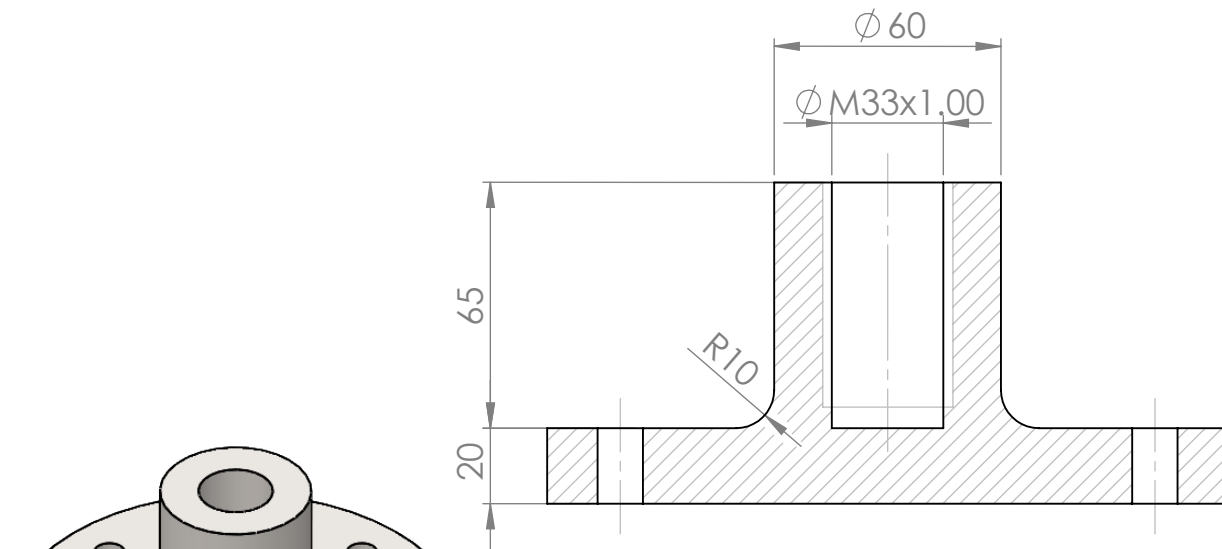
SECCIÓN B-B ESCALA 1 : 2
