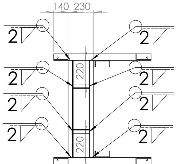
SECCIÓN E-E
