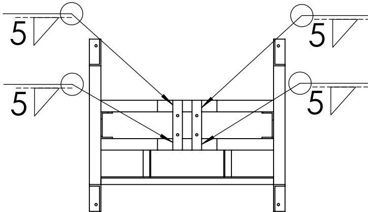
SECCIÓN C-C
