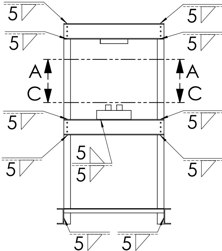
SECCIÓN A-A
