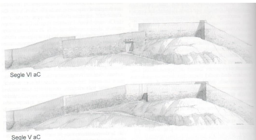
Figura 6. Alçats reconstruïts de les defenses de la zona 2 de Sant Julià de Ramis (Burch, Nolla i Sagrera, 2011, 160).
