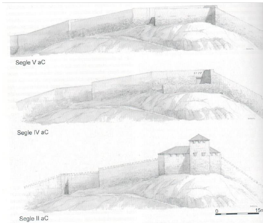
Figura 19. Alçats reconstruïts de les defenses de la zona 2 de Sant Julià de Ramis (Burch, Nolla i Sagrera, 2011, 160).
