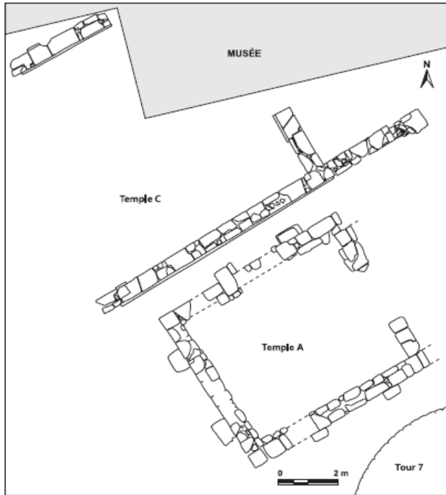
Figura 20. Planta dels temples del Puig de Sant Andreu (Martín et al. , 2010, 99).
