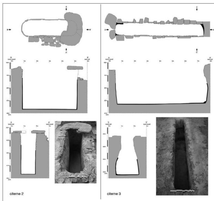
Figura 15. Cisternes 2 i 3 de l'oppidum d'Ullastret (Martín et al. , 2010, 100).
