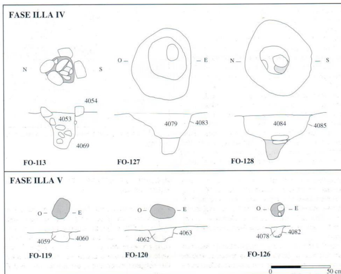
Figura 2. Plantes i seccions dels forats de pal excavats a l'Illa d'en Reixac (Martín, Buxó, López, i Mataró, 1999, 42).
