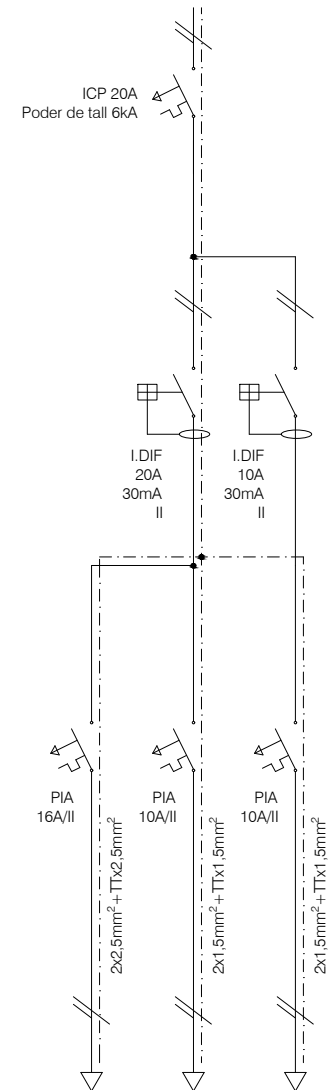
SUBQUADRE HABITACIONS INDIVIDUALS - Línia 16 i línia 4
