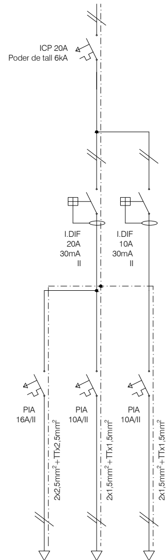
SUBQUADRE HABITACIONS DE MATRIMONI - Línia 4
