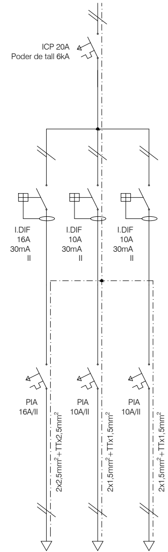
QUADRE ÀTIC - Línia 2
