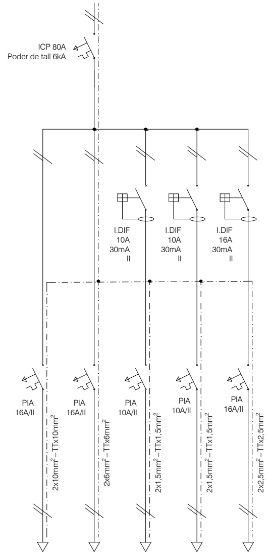
QUADRE PRIMERA PLANTA - Línia 1
