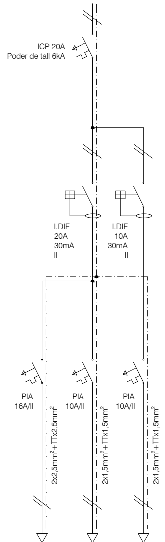
SUBQUADRE SUITE 1,2,3 i 4 - Línia 16
