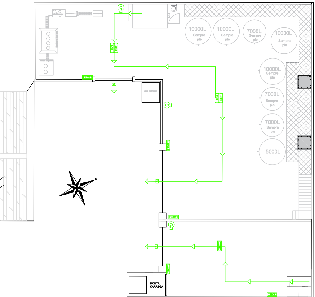
Planta baixa
