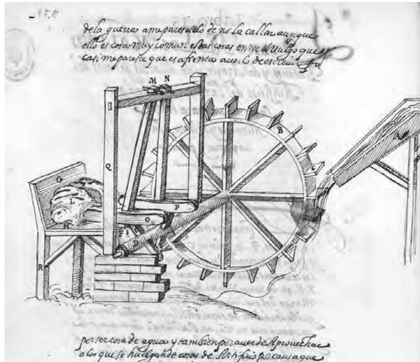
Fig. 1. Dibuix del mecanisme d'un molí draper al segle XVI fet per l'enginyer Pedro Juan de Lastanosa en el llibre manuscrit Los veintiún libros de los ingenios y de las máquinas (còpia posterior del s. XVII). Biblioteca Digital Hispànica.
