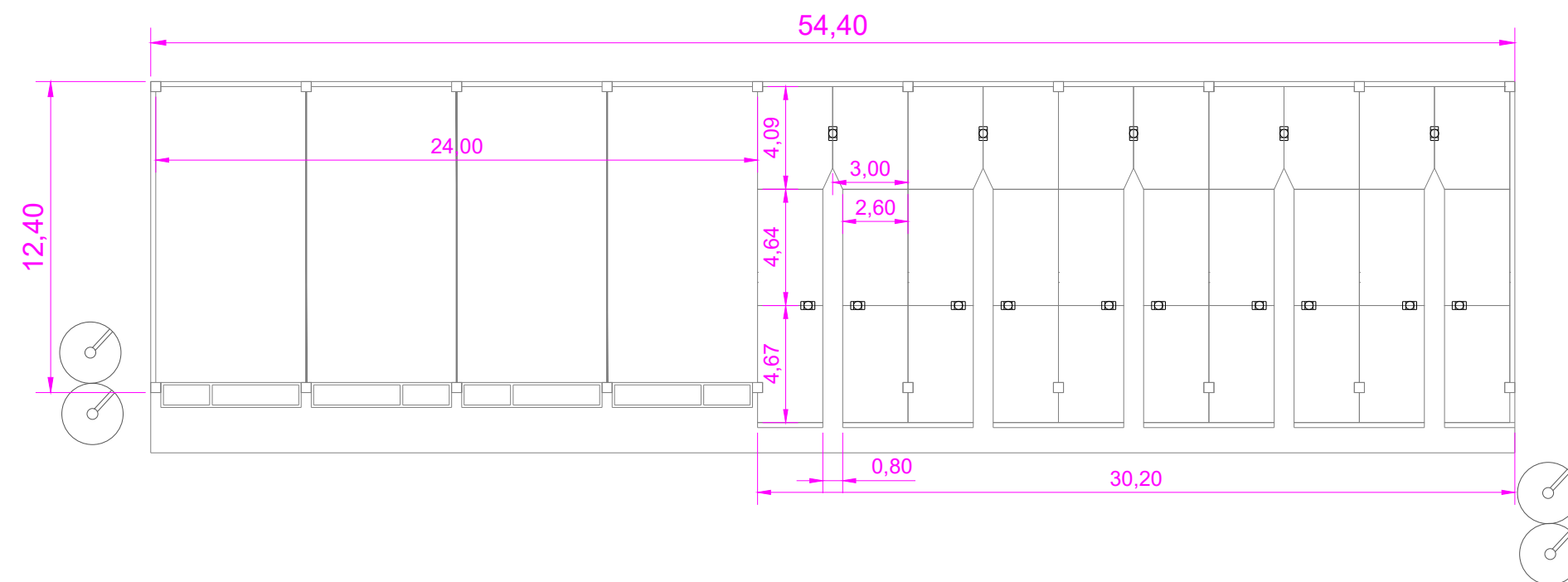
Façana S
