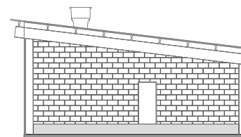
Façana S
