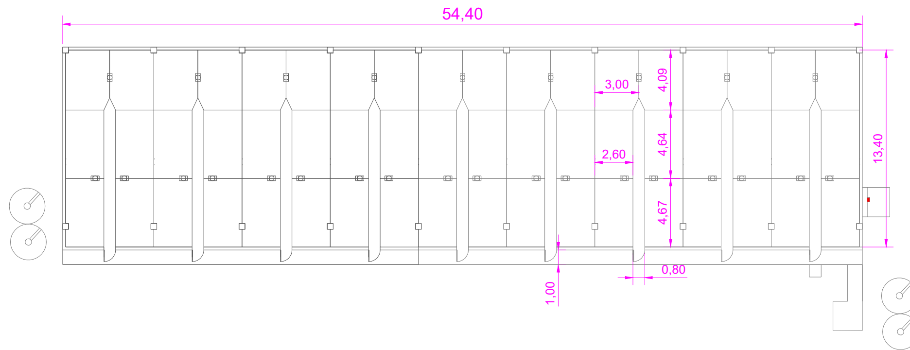
Façana E
