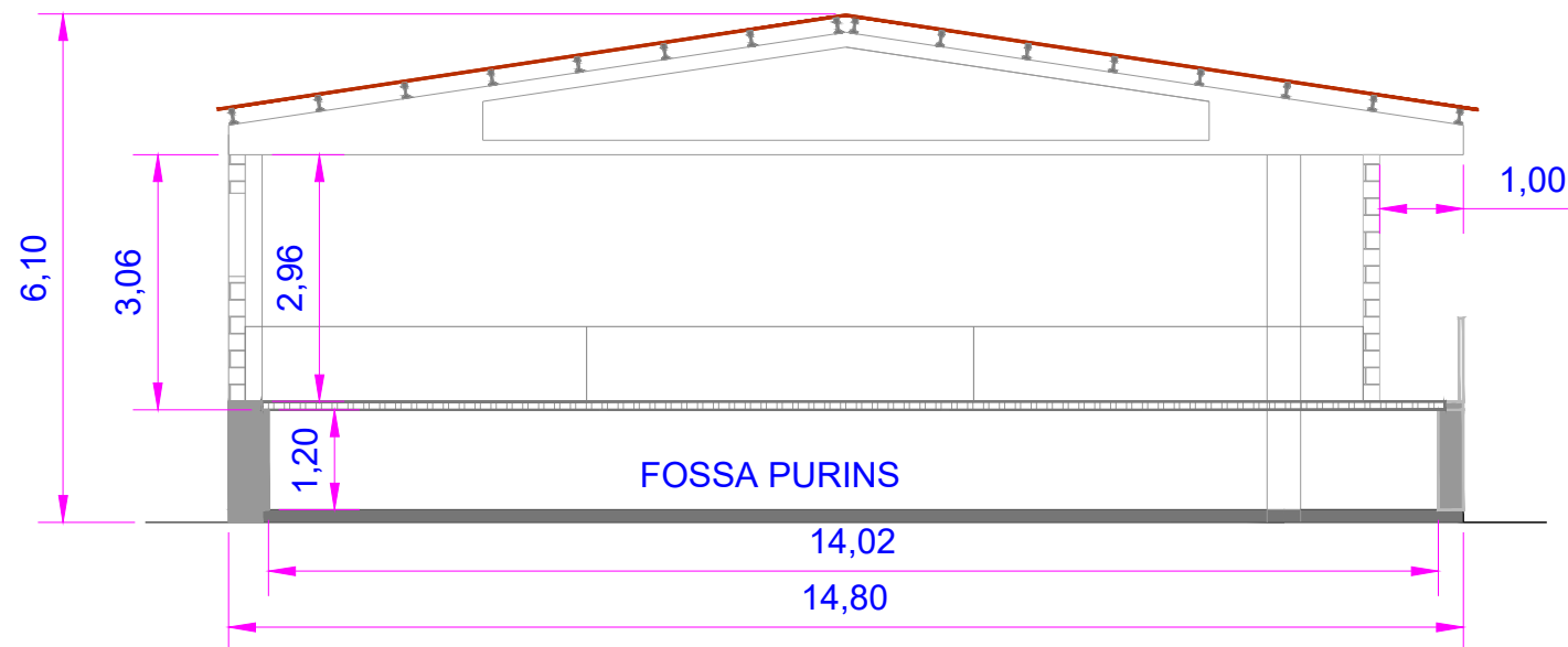
Secció O
