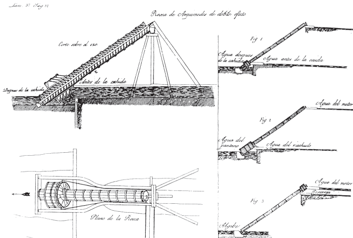
Imatge 4. Rosca d'Arquímedes de doble efecte
