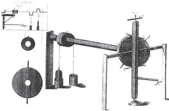
Imatge 11. Màquina ideada per Ametller per a fer pujar i baixar, alternativament, els èmbols de les bombes per treure aigua
