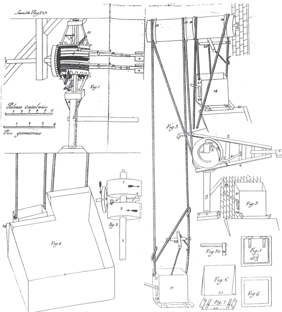
Imatge 12. Màquina de Montiu per extreure aigua d'un pou mitjançant grans recipients cúbics
