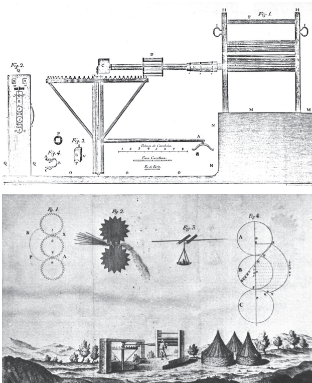
Imatge 1. Màquina de bregar: Vistes esquemàtiques de la màquina de bregar cànem
