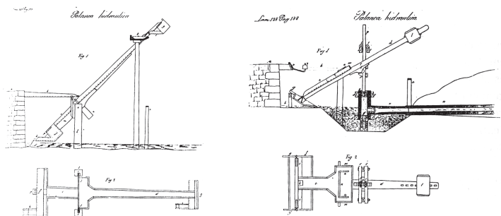
Imatge 5. Palanca hidràulica de Mr. Dublin (esq.). Variant com a motor d'una bomba impel·lent (dreta)
