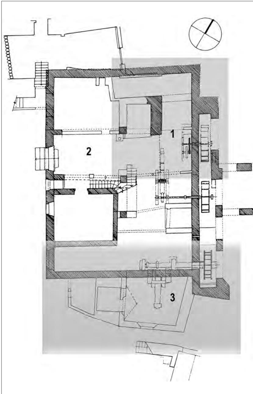
Planta de la Farga d'aram de Banyoles. Dibuix: J. Moner. 1. Primer edifici del Comú de 1685 amb un sol martinet. 2 Farga d'en Bernich del segle XVIII. 3. Possible ampliació de la segona meitat del segle XVIII.
