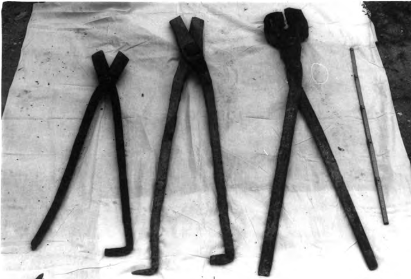
Tenalles de fargaire la Farga d'aram de Banyoles pertanyents a una col·lecció particular. Autor: E. Palmada.
