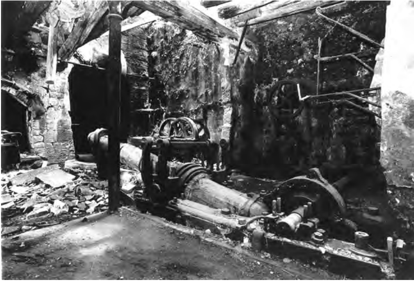
El martinet de batre de la Farga d'aram de Banyoles els anys 80 del segle XX (CRDI).
