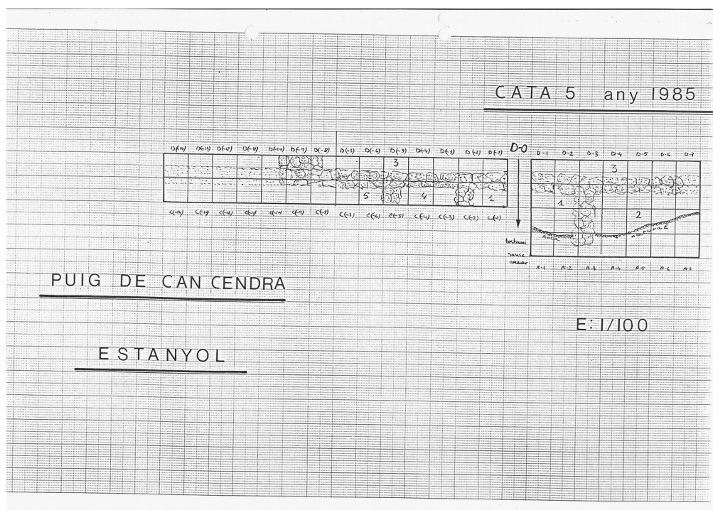
Figura 43: Dibuix general en planta de la Cata 5 el 1985. Font: Arxiu MAC-Girona.
