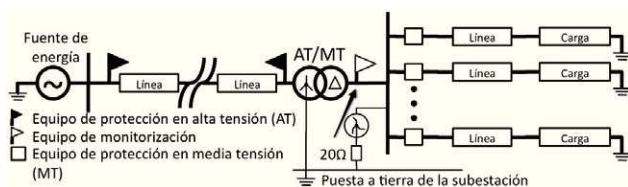
Figura 3. Diagrama unifilar de las subestaciones de distribución donde se registraron los eventos reales.
