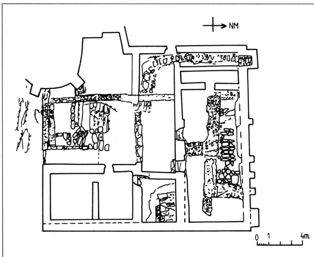
Fig. 3. Planta general del palau de l'abat (dibuix de J. Burch i F. Tió).
