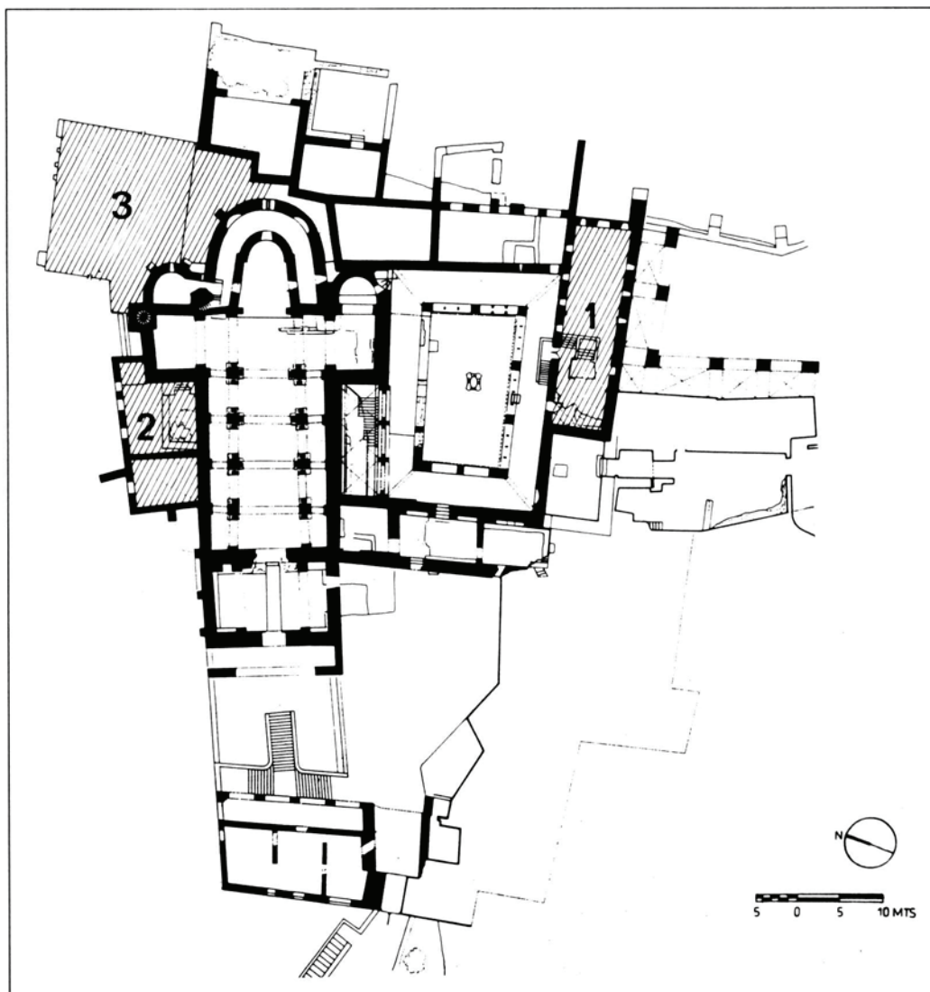
Fig. 2. Planta general del conjunt arquitectònic de Sant Pere de Rodes (basada en la de J. A. Martínez, 1980): 1) refectori; 2) sagristies noves; 3) palau de l'abat.
