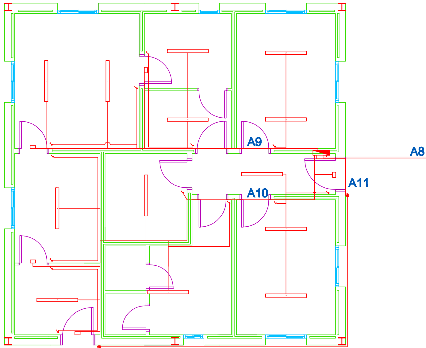
INSTAL·LACIÓ ELÈCTRICA D'ENLLUMENAT
