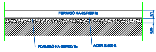
DETALL DE LA PAVIMENTACIÓ
