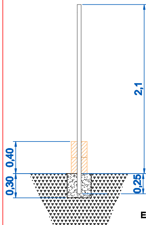
DETALL D' UNIÓ DE LA CIMENTACIÓ AMB ELS PALS DE LA TANCA PERIMETRAL
