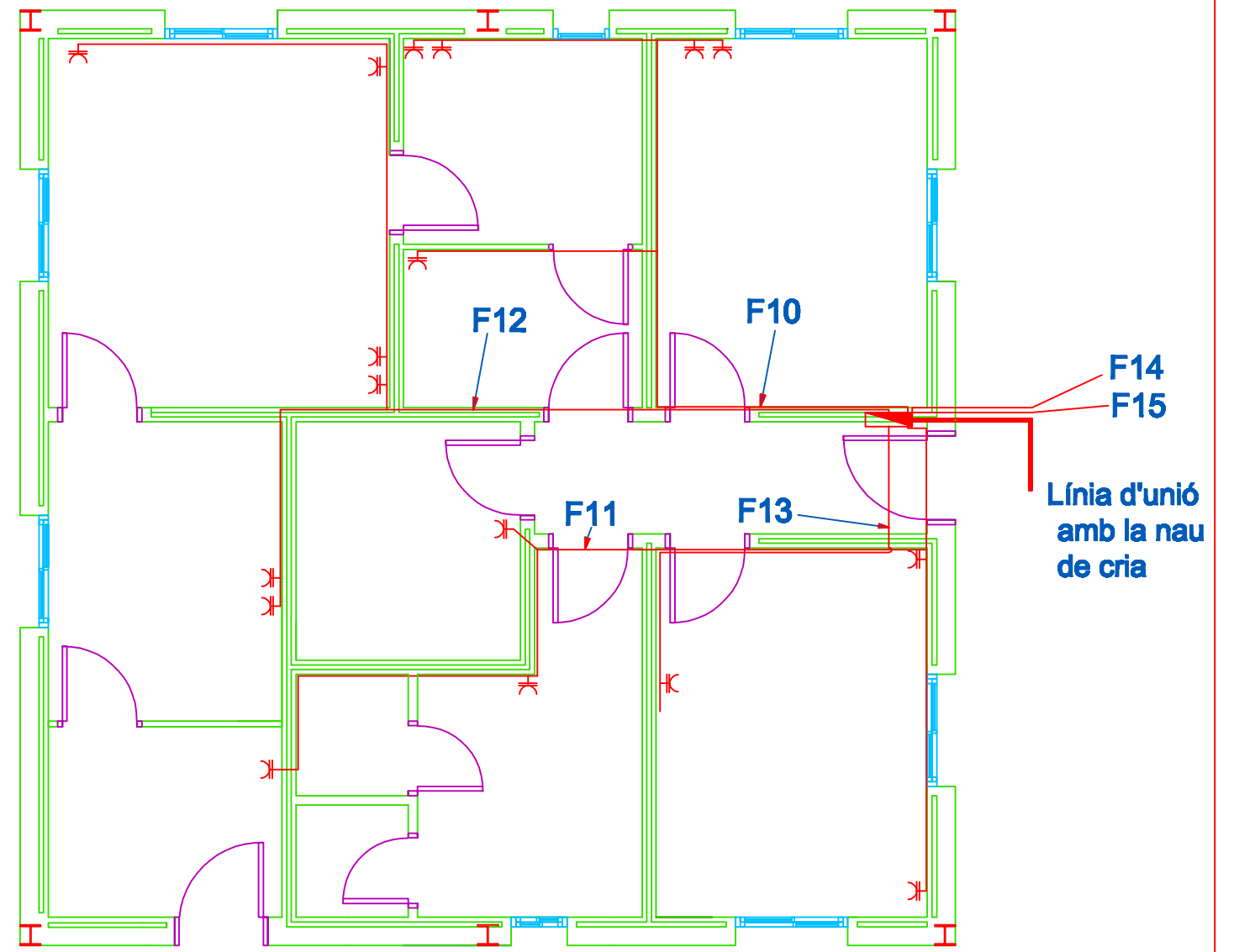
INSTAL·LACIÓ ELÈCTRICA DE FORÇA
