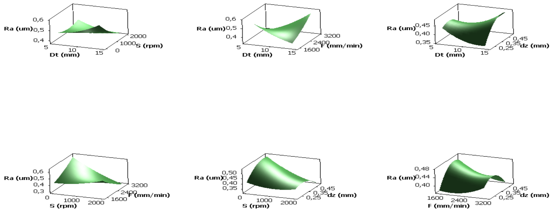
Figura C.4 Superfícies de resposta per la rugositat superficial de l'anàlisi preliminar
