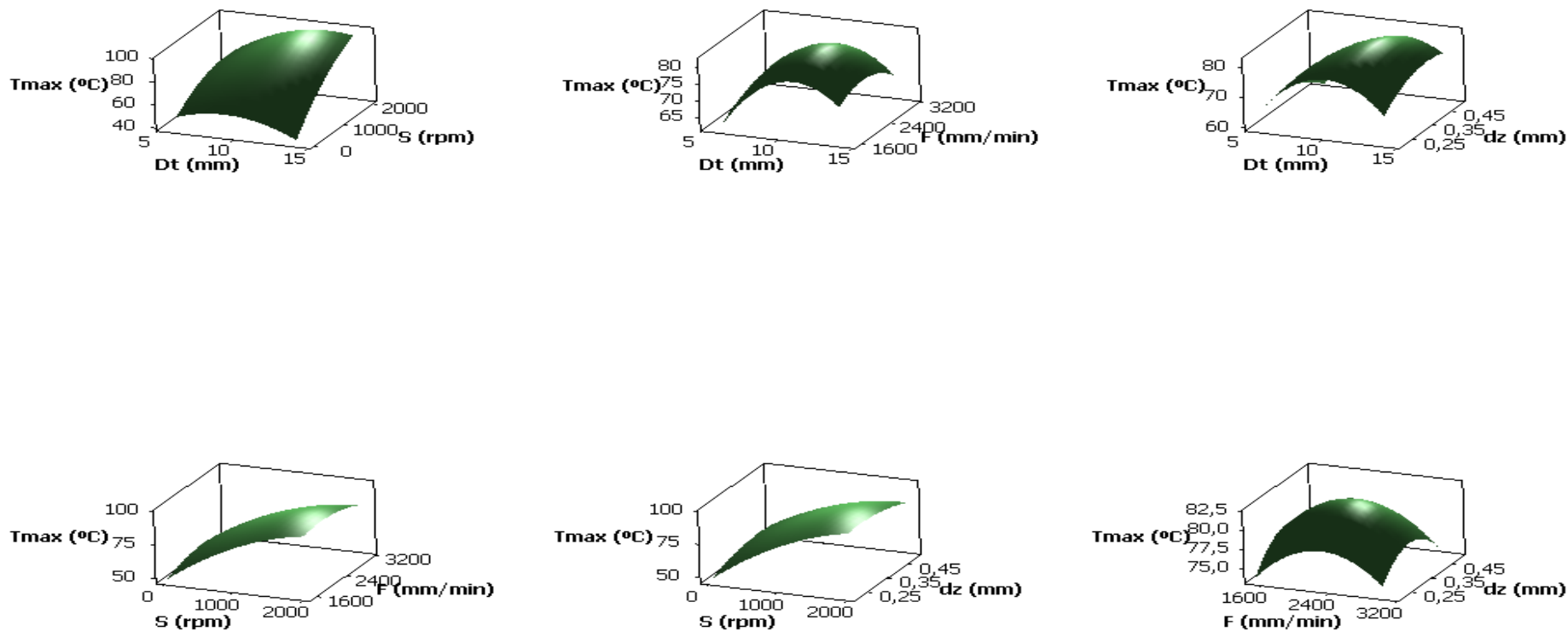
Figura C.3 Superfícies de resposta per la temperatura màxima de l'anàlisi preliminar
