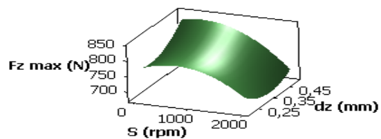
Figura C.2 Superfícies de resposta per la força màxima de l'anàlisi preliminar
