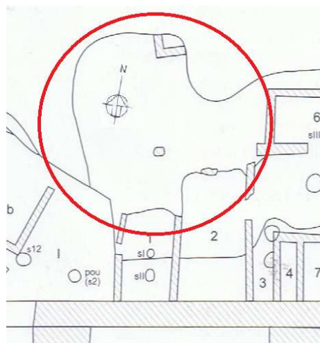
Fig.4.19.1.: Planta de detall de la zona davant de la porta i cambres 1 i 2. Extret de: Pere de Palol, El Castrum del Puig de les Muralles de Puig Rom . Girona: 2004, p. 39
