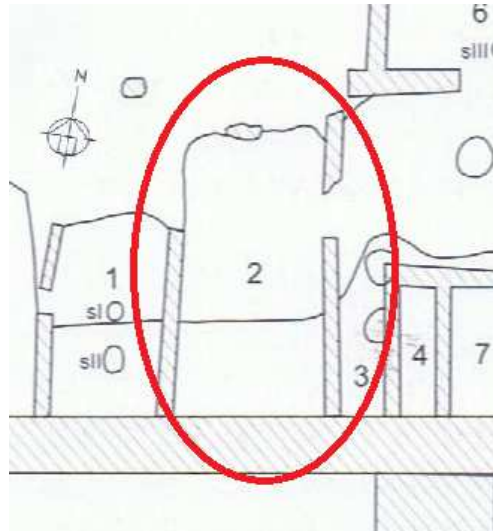
Fig.4.23.1.: Planta de detall de la cambra 2. Extret de: Pere de Palol, El Castrum del Puig de les Muralles de Puig Rom . Girona: 2004, p. 39
