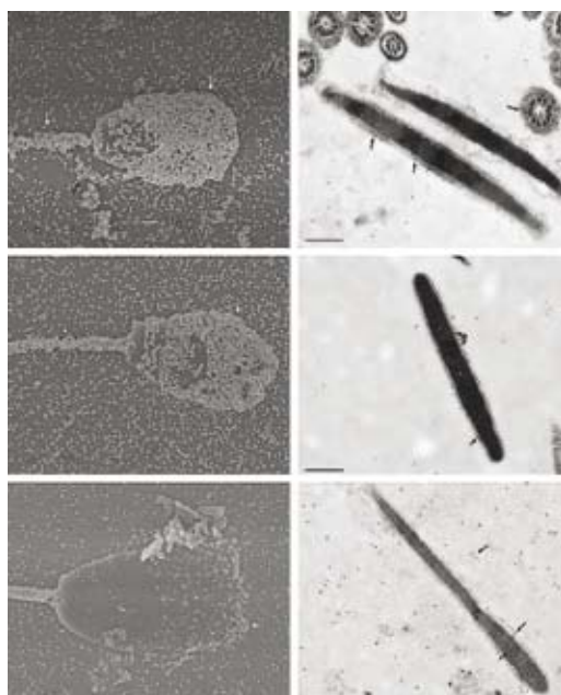
Fig.10. Inmunoglod para GLUT-3 para SEM (izquierda) y TEM (derecha). Imagen superior: Semen fresco; Imagen media: semen refrigerado a 5°C; Imagen inferior: semen descongelado (Sancho et al, 2007).
