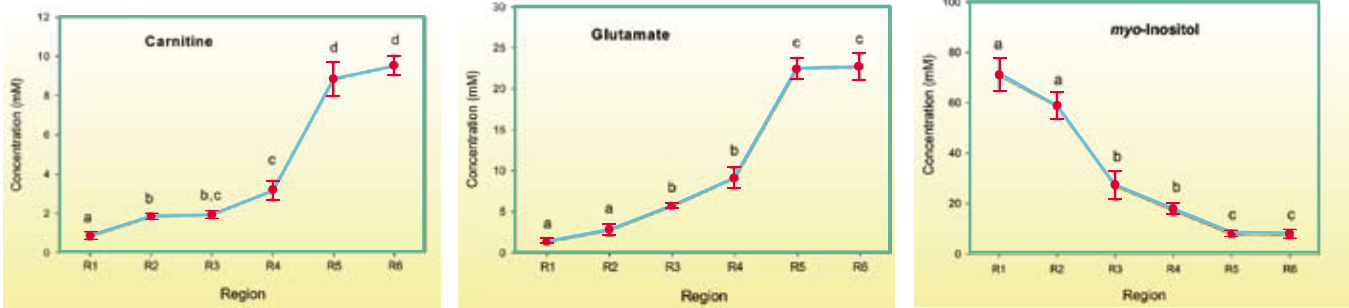
Fig.7. Gráficas que muestran las variaciones en la concentración de Carnitina, Glutamato e Inositol en el fluido epididimario a lo largo de sus 6 subregiones (Pruneda et al., 2006, 2007).
