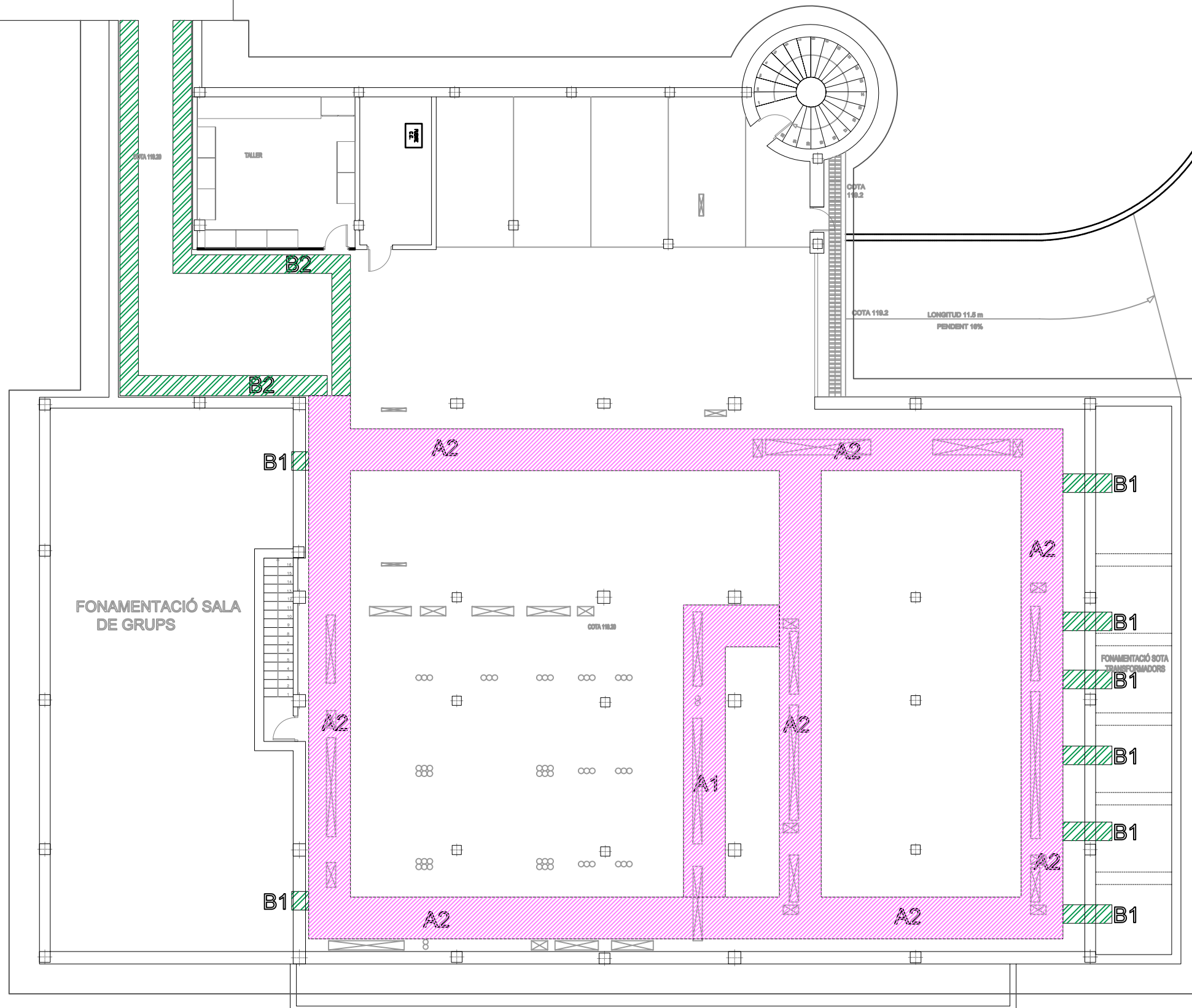
PLANTA SOTERRANI
