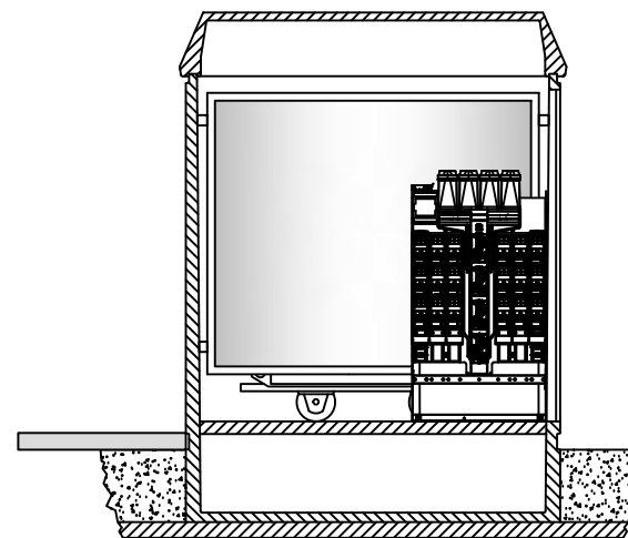
SECCIÓ B-B'
