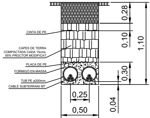
2 CIRCUITS EN CALÇADA AMB 2 TUBS FORMIGONATS
