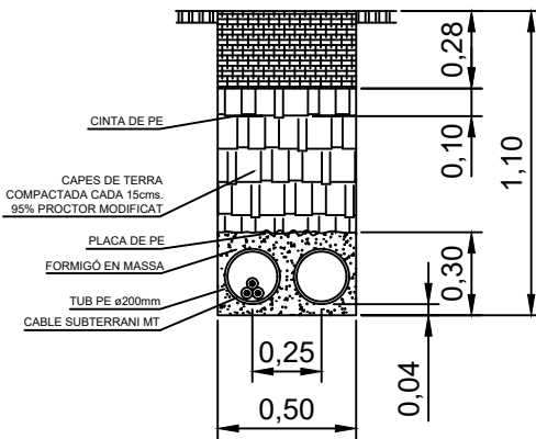
1 CIRCUIT EN CALÇADA AMB 2 TUBS FORMIGONATS
