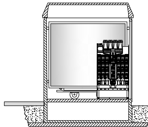
SECCIÓ B-B'
