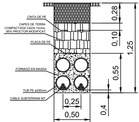
2 CIRCUITS EN CALÇADA AMB 4 TUBS FORMIGONATS
