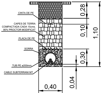
1 CIRCUIT EN CALÇADA AMB 1 TUB PE SEC
