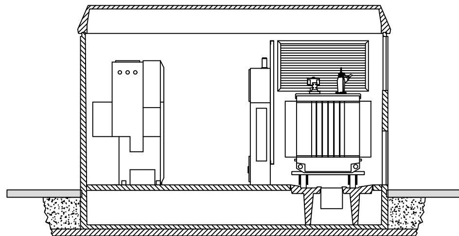
SECCIÓ A-A'
