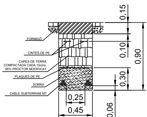
2 CIRCUITS EN VORERA
